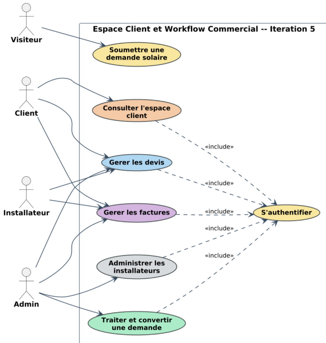
FIGURE 4.7. Diagramme de cas d'utilisation global – Itération 5
