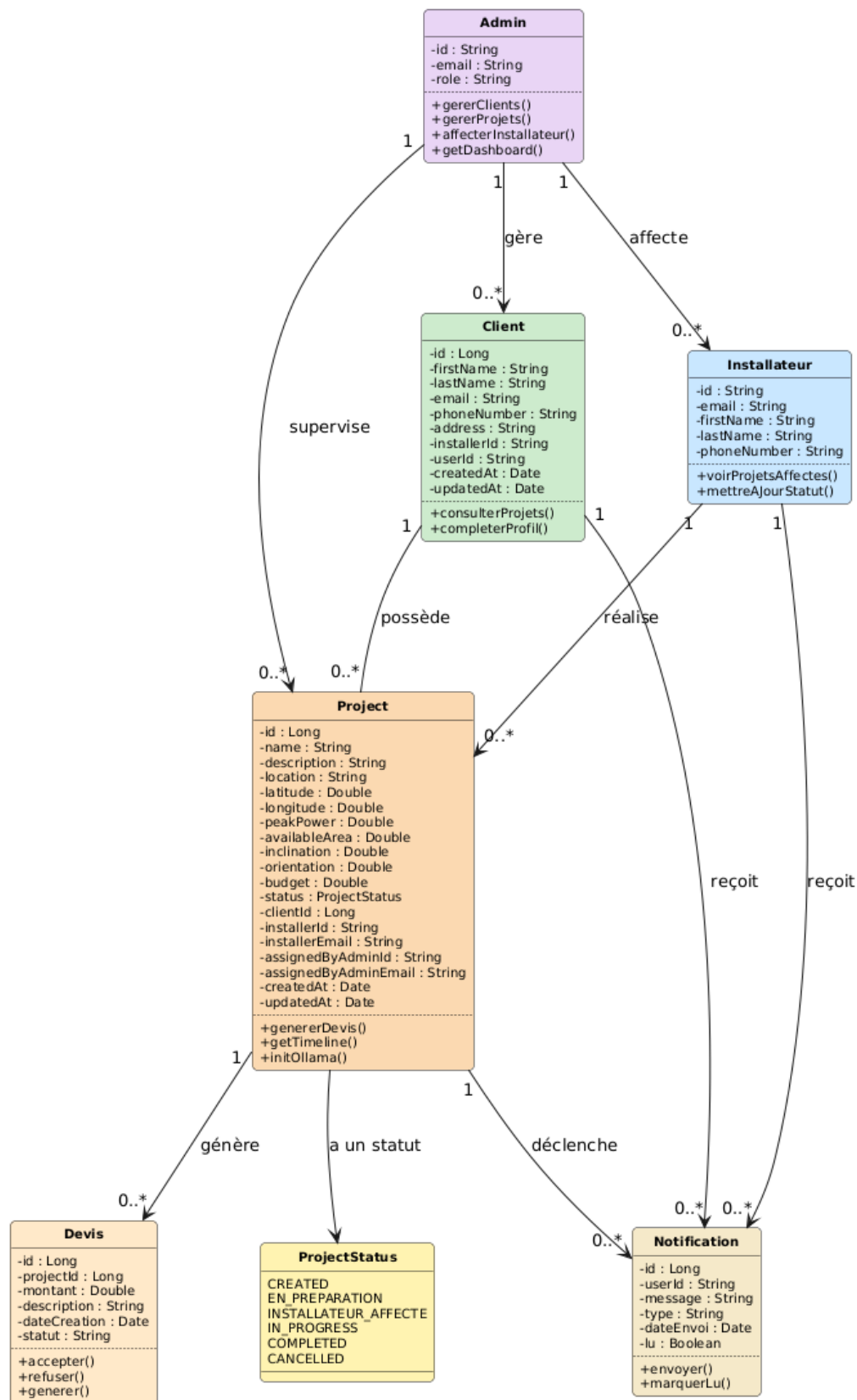
FIGURE 3.9. Diagramme de classes – Itération 2
