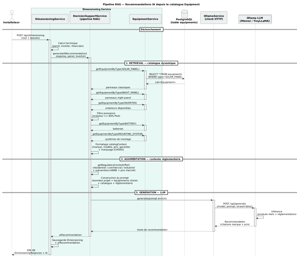
FIGURE 3.20. Diagramme de séquence du pipeline RAG
