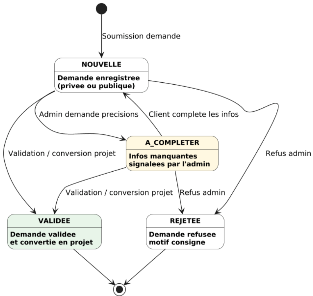
FIGURE 4.10. Automate d'états d'une demande solaire
