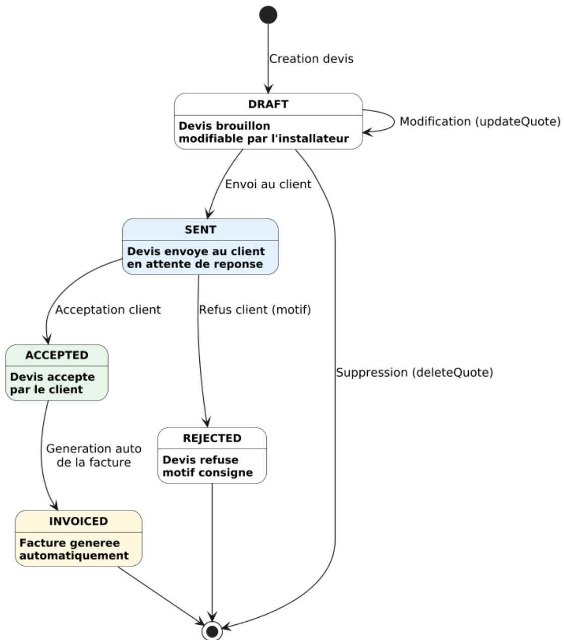
FIGURE 4.9. Automate d'états d'un devis SolarEase
