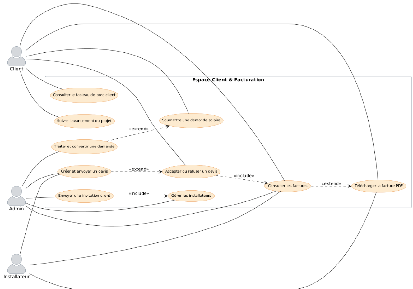
FIGURE 3.13. Diagramme de cas d'utilisation global relatif à l'itération 3
